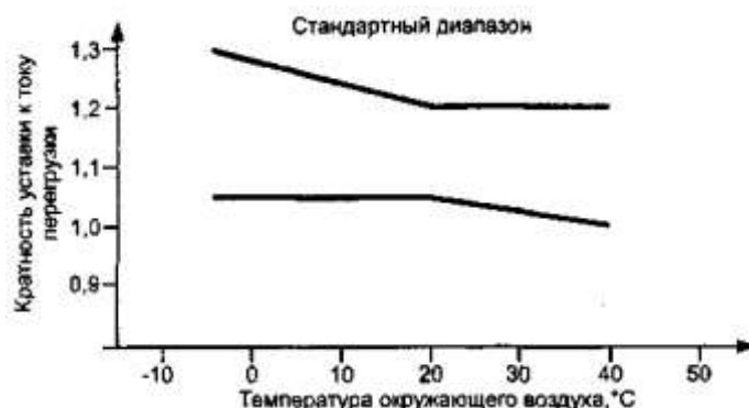
Рисунок 7 — Зависимости пределов кратности уставок тока от температуры окружающего воздуха для компенсированных реле перегрузки с выдержкой времени (см. 7.2.1.5.1)
