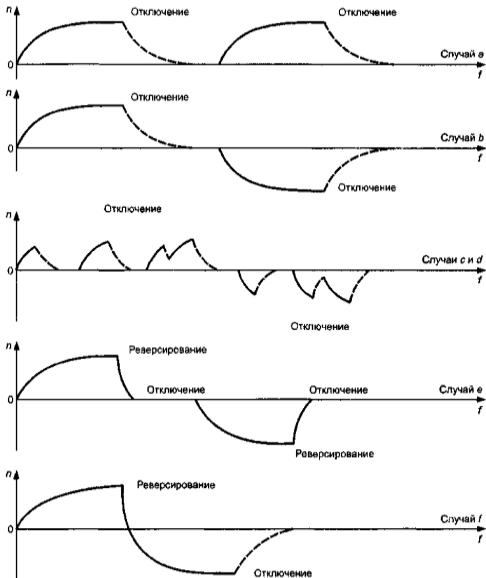
Рисунок 6 — Примеры кривых скорость — время, соответствующие случаям а)–f) по 4.3.5.5 (пунктирные участки кривых обозначают периоды обесточивания двигателя)
